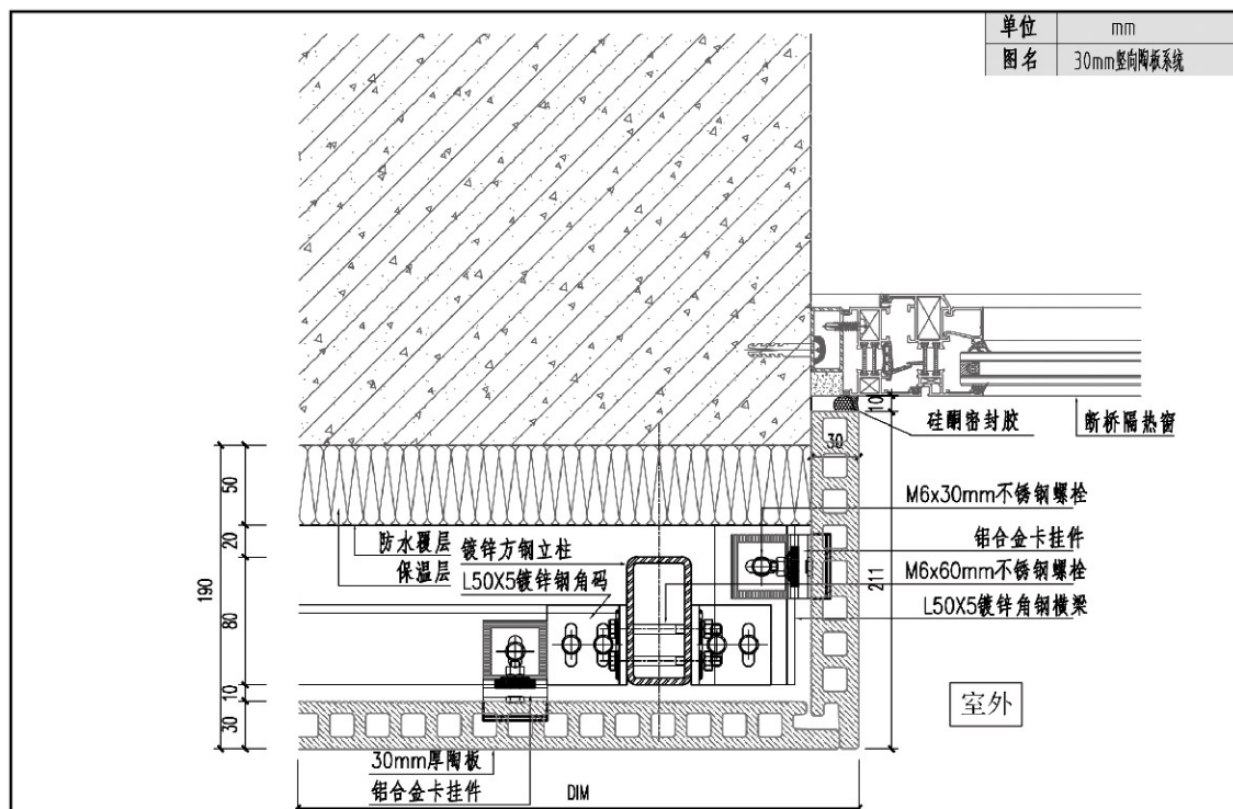
陶板幕墙窗侧节点图(陶板收口)
