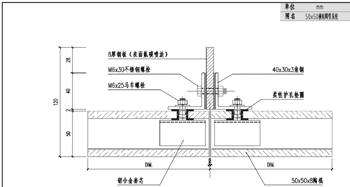
横剖节点图
