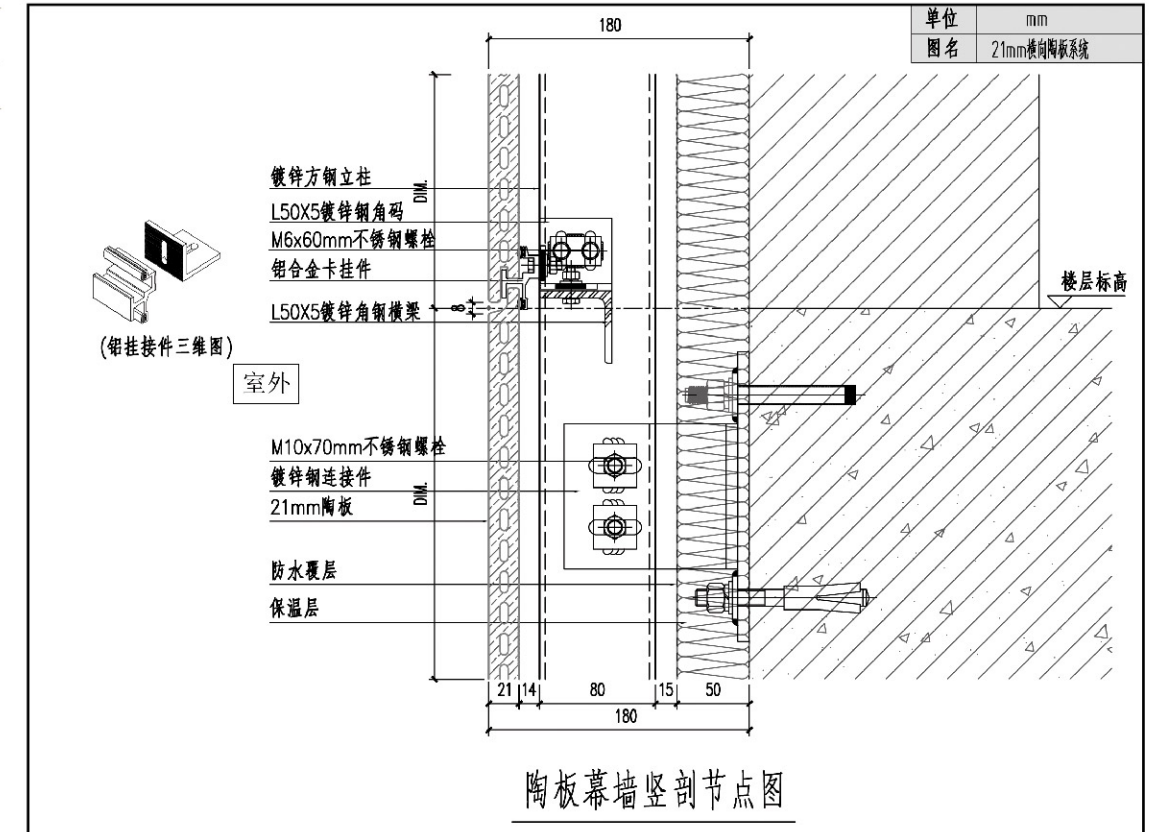
21mm 陶板系统 安装节点图
