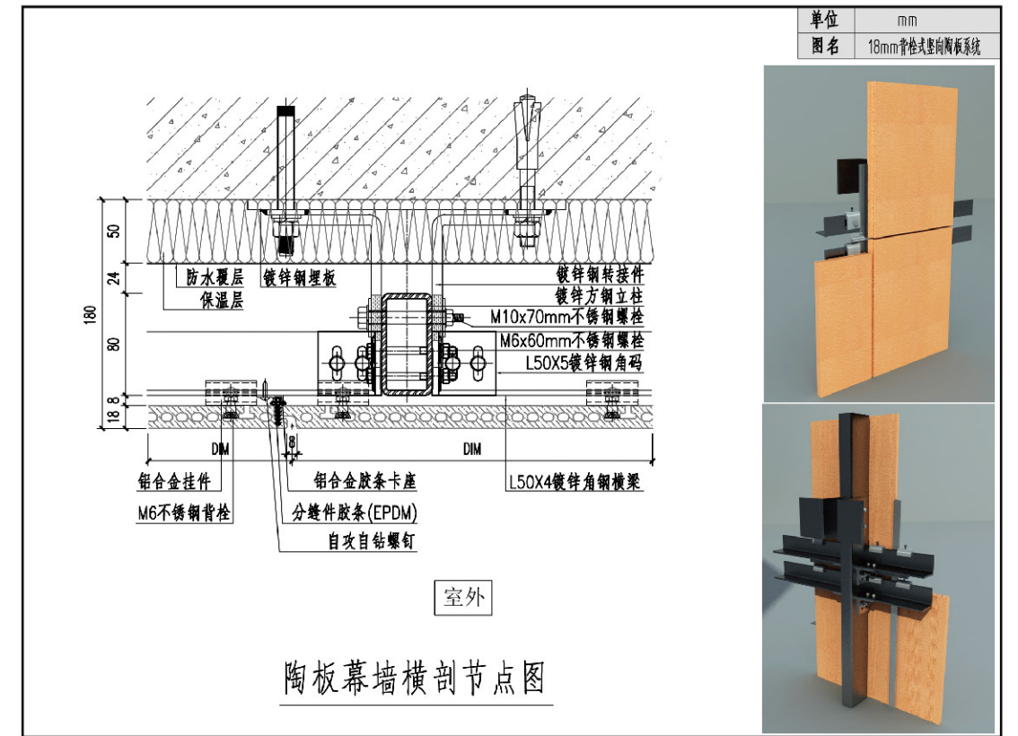
4. 18mm 背栓式竖向 系统安装节点图
