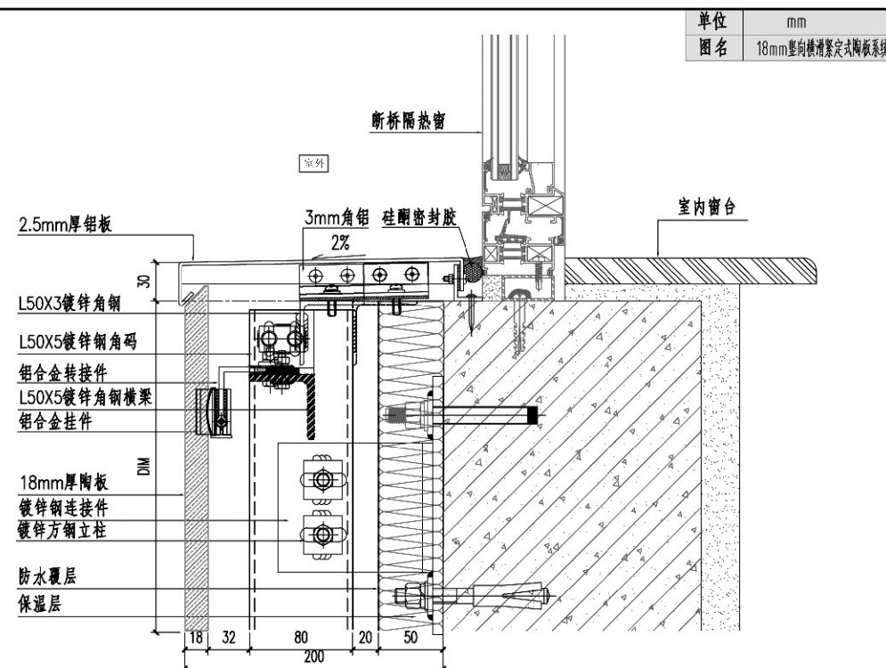
陶板幕墙窗下口节点图(铝板收口)
