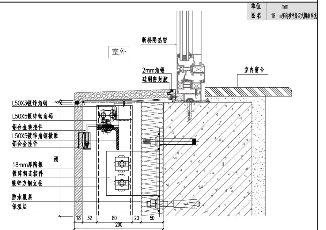
陶板幕墙窗下口节点图(陶板收口)
