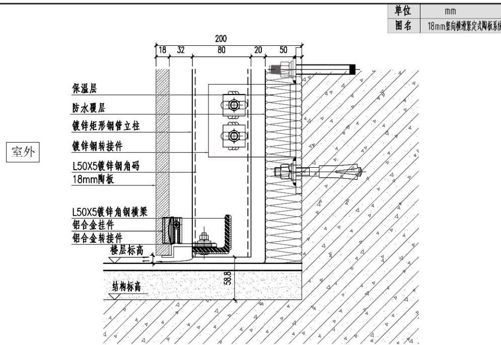
陶板幕墙起底节点图
