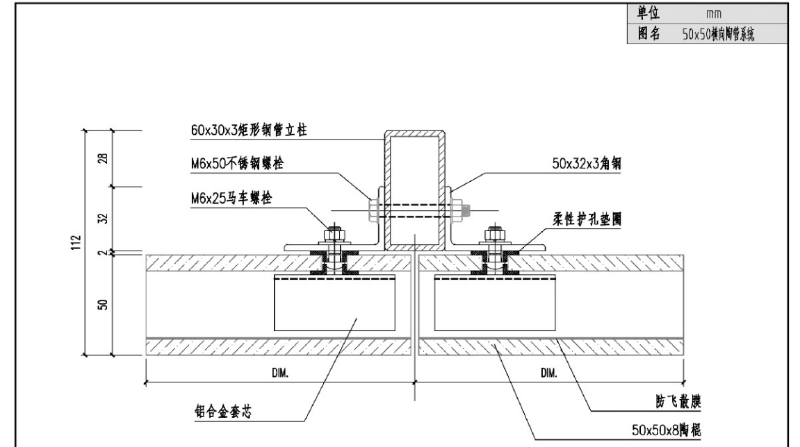
横剖节点图
