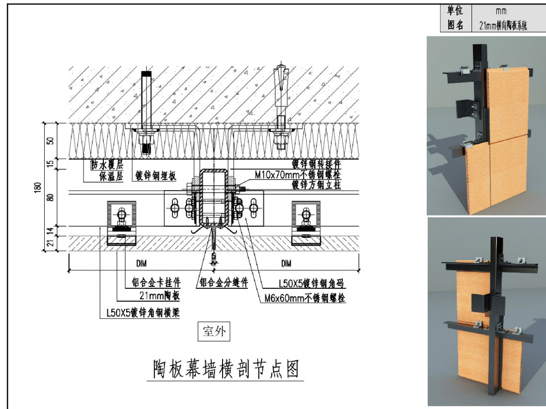
21mm 陶板系统 安装节点图
