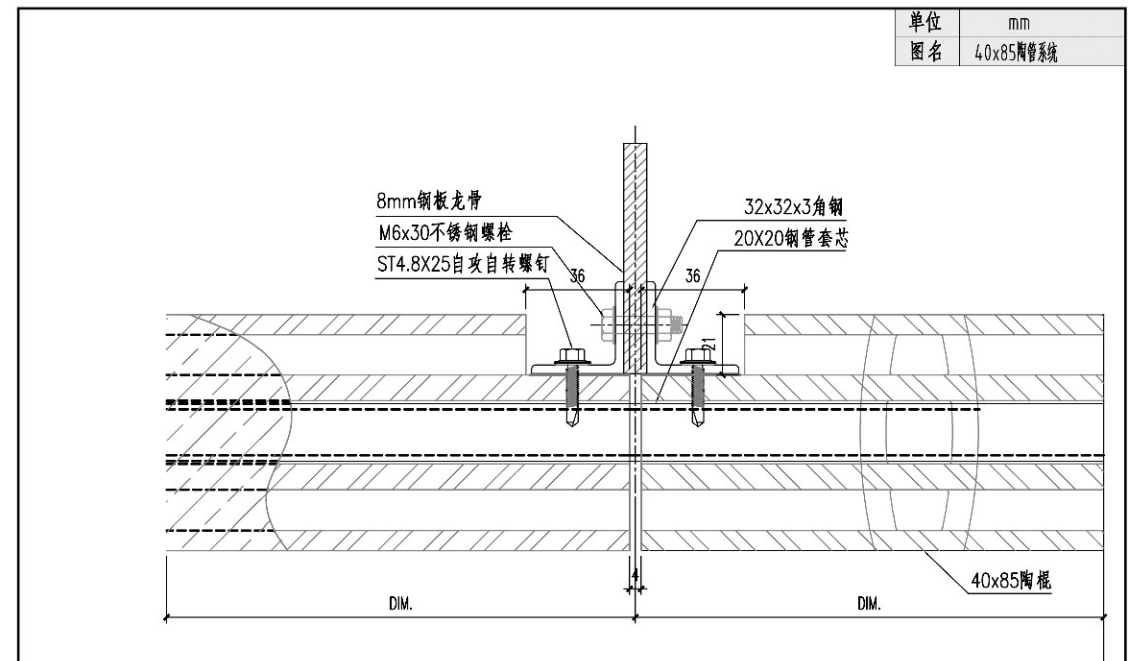
横剖节点图
