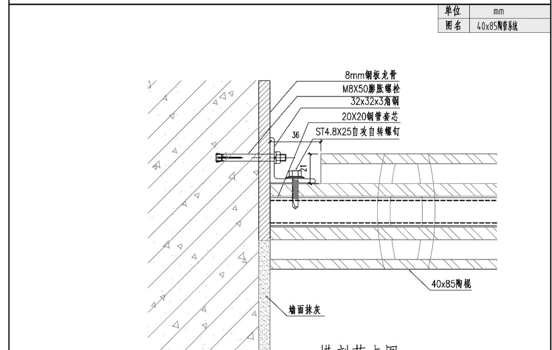
横剖节点图
