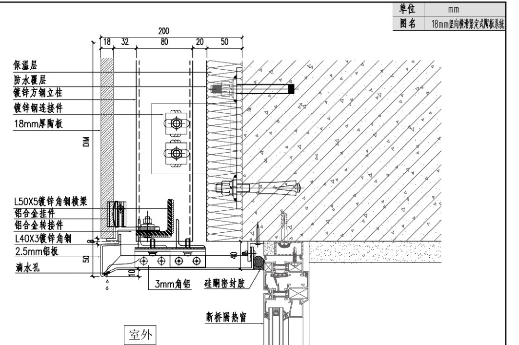
陶板幕墙窗上口节点图(铝板收口)
